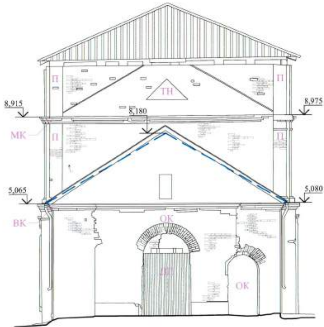
Западный фасад
