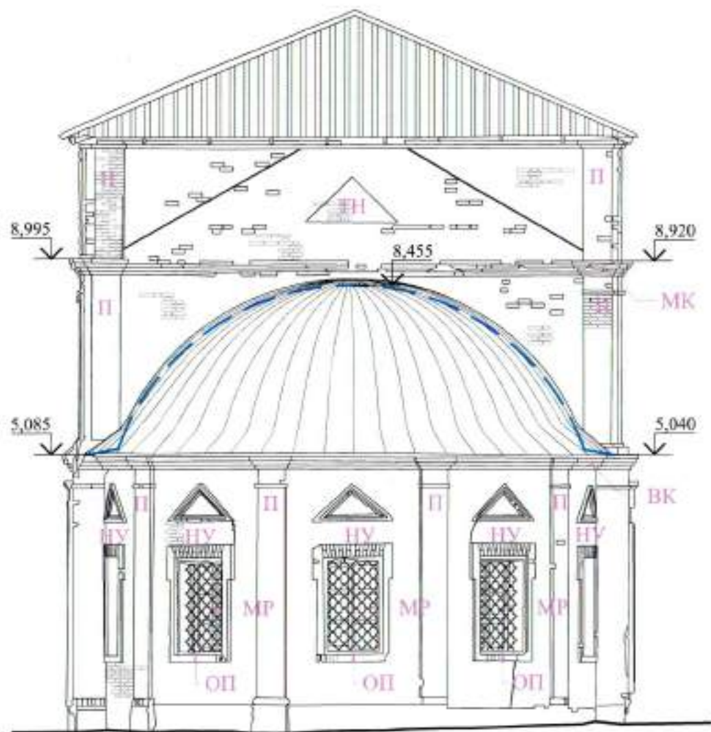
Восточный фасад
